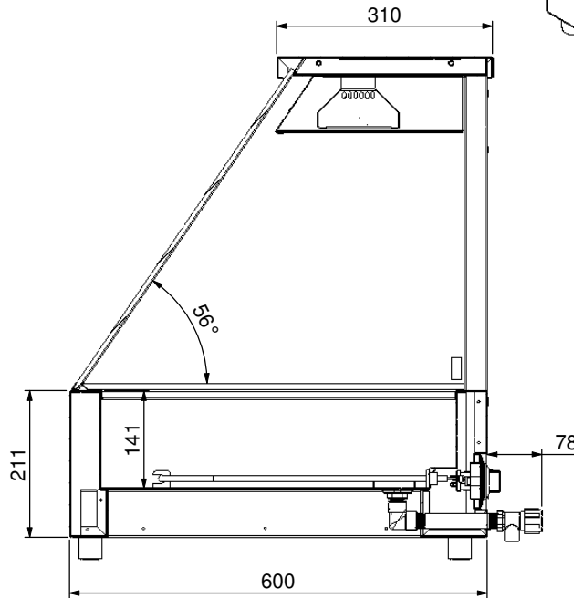
SECTION CJ-CJ
